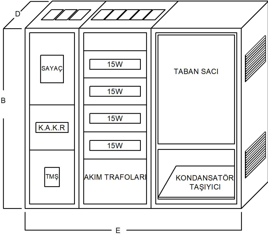
Perde Görünüş
